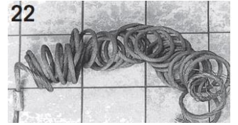
22 Pokud se ocelové lano táhne přes ostré hrany, má sklon se v nezátíženém stavu navíjet.
