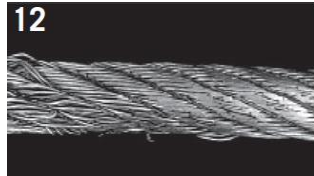
12 Příliš široký kladkostroj špatně podepírá ocelové lano. Následkem je rychlé zlámání drátů na styčném povrchu.
