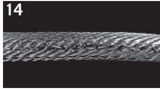
14 Toto nekroutové ocelové lano bylo taženo přes okraj kladkostoje, a tím se hodně poškodilo.
