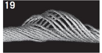
19 Vznik košíku na nekroutivém ocelovém laně. Pokud jste viděli jedno, viděli jste všechny.
