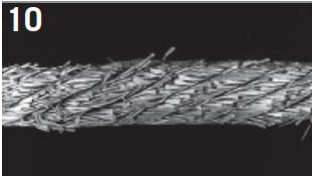
10 Toto ocelové lano pracovalo v příliš úzkém kladkostí.
