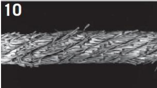
10 Toto ocelové lano pracovalo v příliš úzkém kladkostroji.
