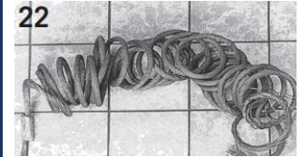
22 Pokud se ocelové lano táhne přes ostré hrany, má sklon se v nezatíženém stavu navíjet.
